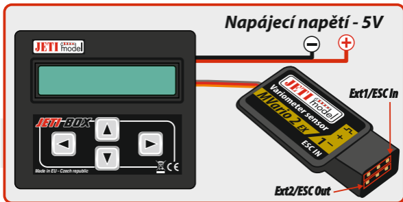
Obr. 1: Zapojení MVaria2 k Jetiboxu
