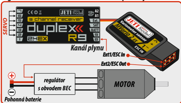
Obr. 5: Připojení MVario2 do vstupu přijímače
