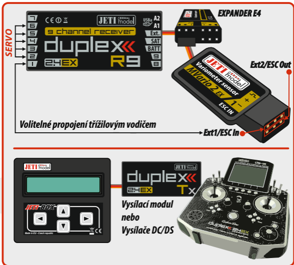
Obr. 3: Zapojení MVario2 prostřednictvím Expanderu
