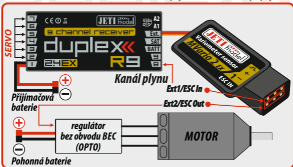
Obr. 6: Připojení MVario2 do vstupu přijímače s přijímačovou baterií
